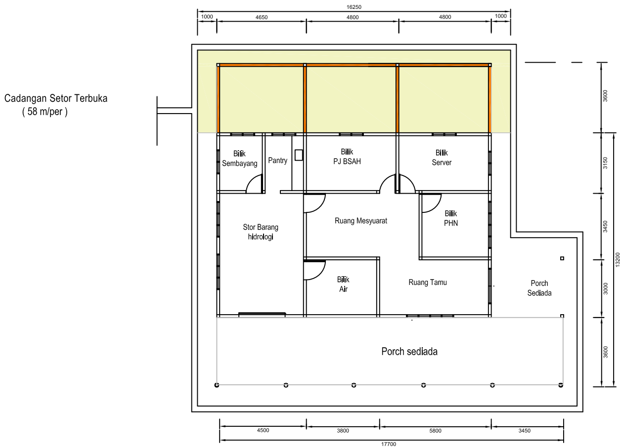
Pelán Rasuk Bumbung
